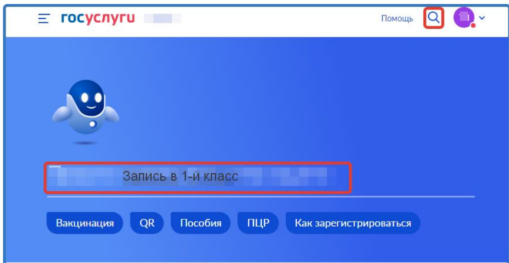
Рисунок 2 – Поиск услуги
